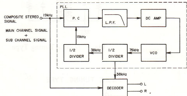
Fig. 11 MPX IC Function
