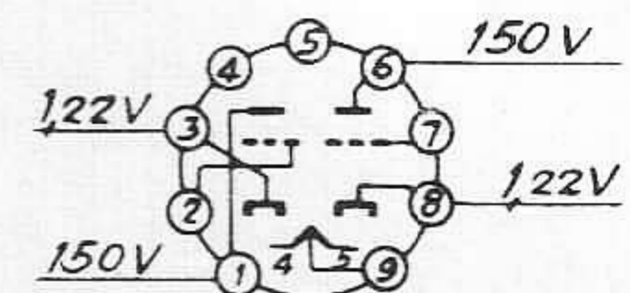
ECC83
