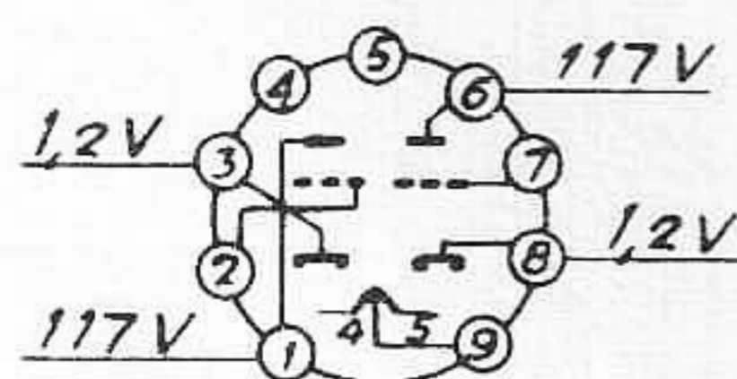
ECC83
