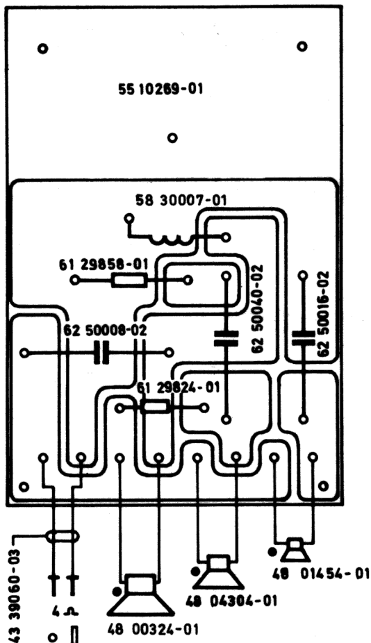
KOPPLINGSSCHEMA
