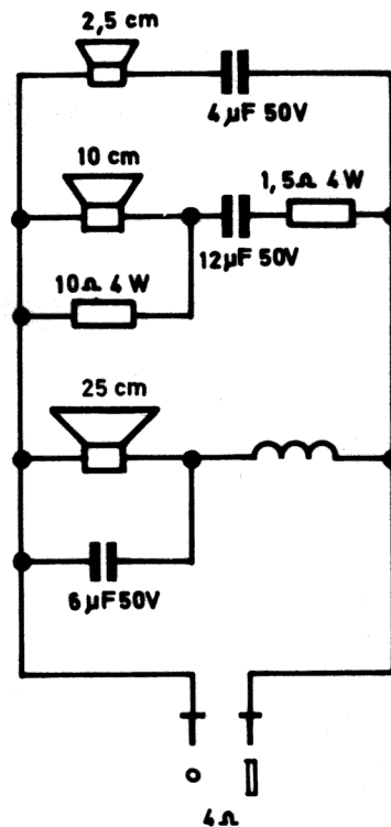
SCHALTSCHEMA
