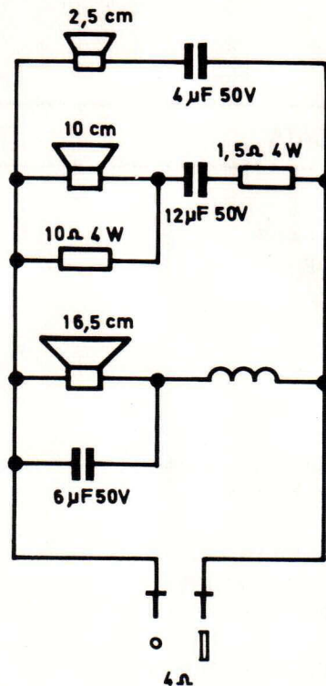
SCHALTSCHHEMA
