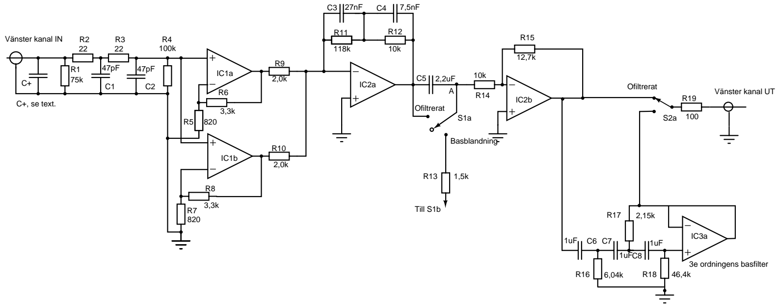
Fig 2. RIAA-stegets kopplingschema. OBS att strömförsörjning och avkopplingskomponenter inte visas.
