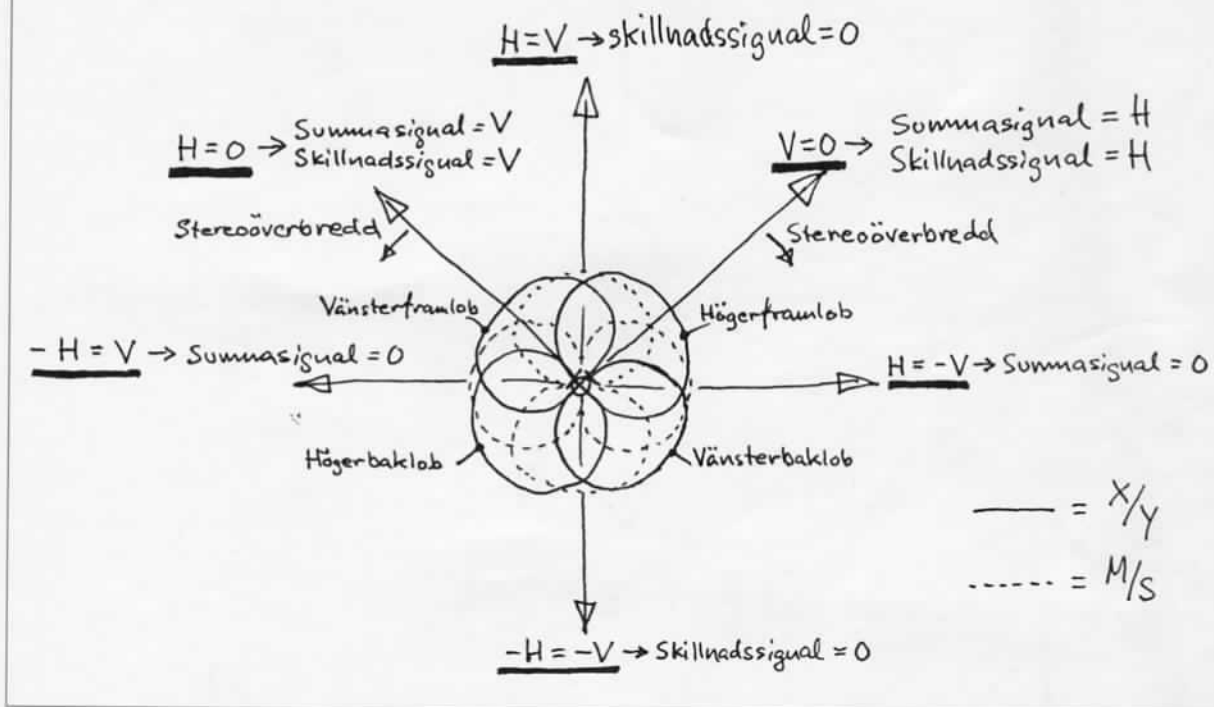
Fig. 1: Här ser man hur en X/Y- eller M/S-mikrofon (streckad) ser på sin omvärld och kodar den till Höger & Vänster kanal. Notera gärna att varken X/Y eller M/S (med 8-mikrofoner) kan skilja på framåt och bakåt! Det som kodas som "bakljudsbild" är i stället det som faller in från sidorna. Dessutom är det bakifrån infallande ljudet omkastat höger-vänster! Används X/Y blir höger=X, vänster=Y. Används M/S blir höger=M+S, vänster=M-S.
