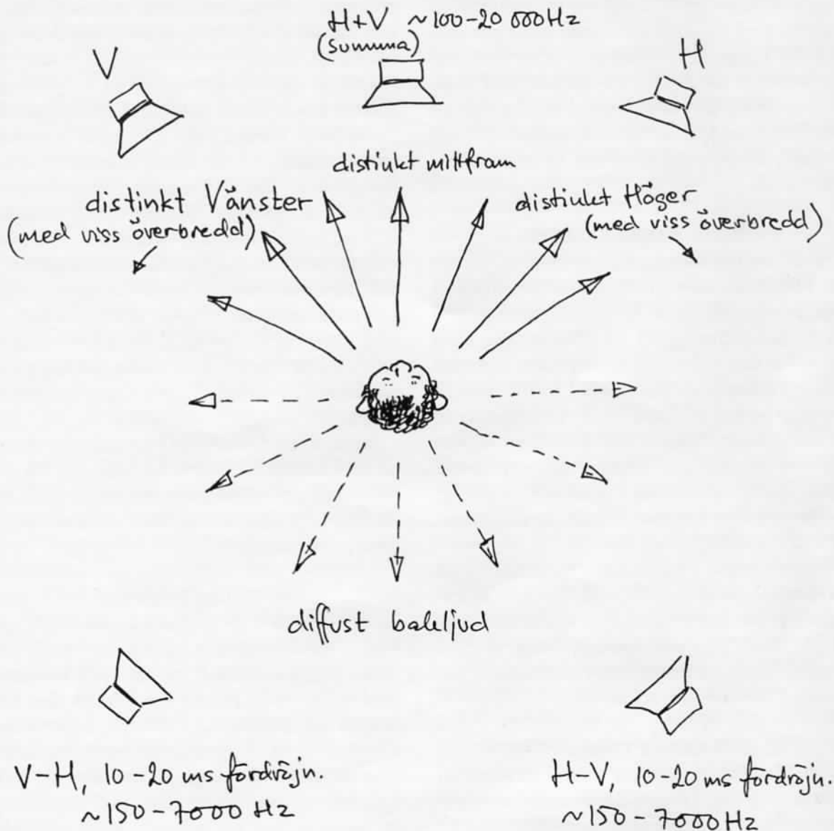
Fig. 5: Med fördröjda och filtrerade bakkanaler får vi det bästa från två världar. En mycket distinkt ljudbild (som t.o.m. sträcker sig utanför framhögtalarna med god precision), en jämn övergång till den lagom diffusa bakljudsbilden och en mycket god okänslighet för lyssnarens placering om man använder mitthögtalare. Bakkanalerna kan även kompletteras med en dipol, siktande åt sidorna, placerad mitt bak.
