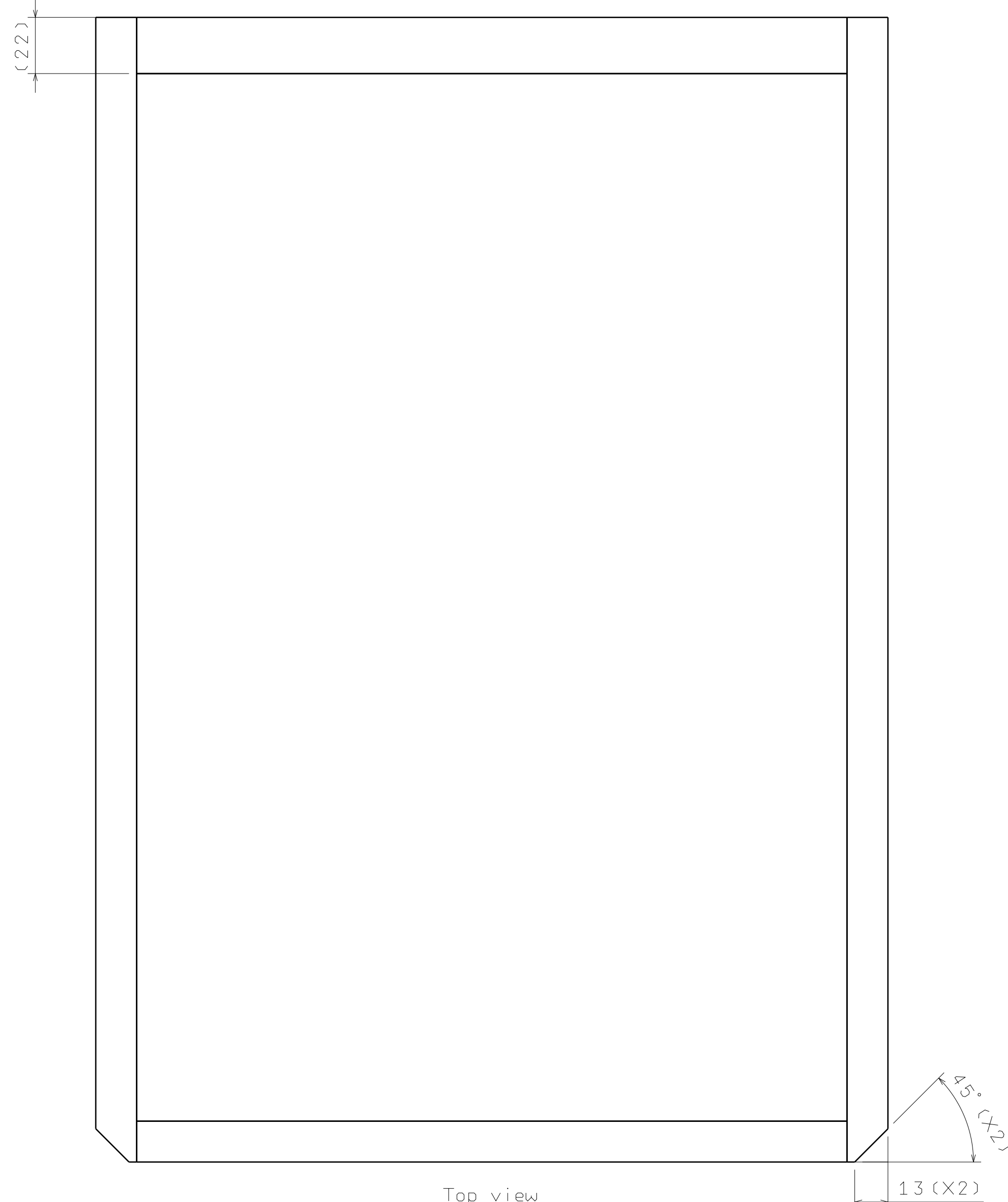
Top view Scale: 2:3
